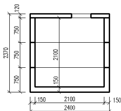
ŘEZ B-B'
