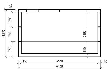
ŘEZ B-B'
